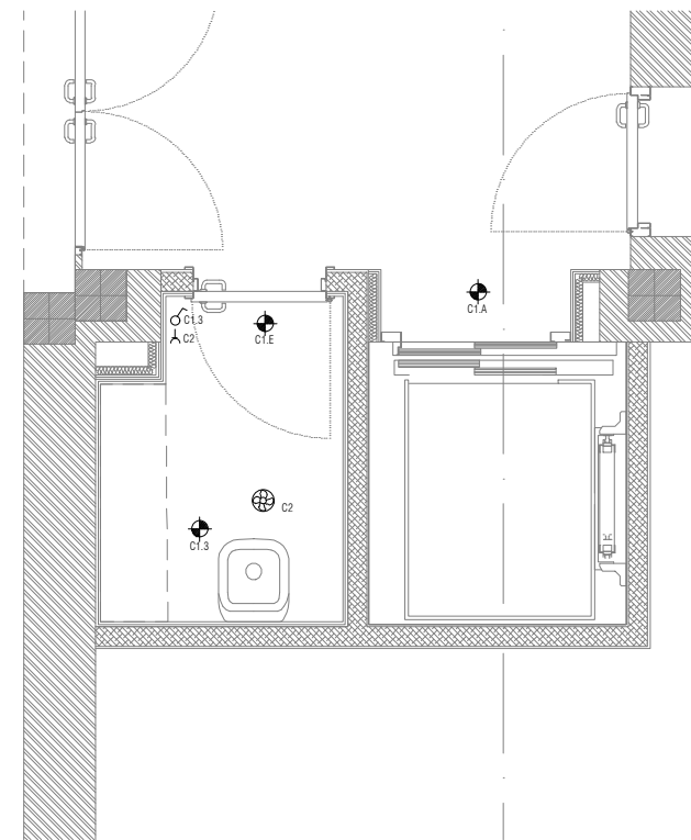
ELECTRICIDAD PLANTA PRIMERA
