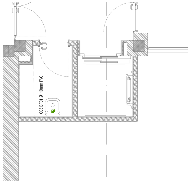
SANEAMIENTO COLGADO Y EMPOTRADO PLANTA PRIMERA
