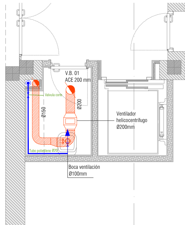
FONTANERÍA Y VENILACIÓN PLANTA PRIMERA
